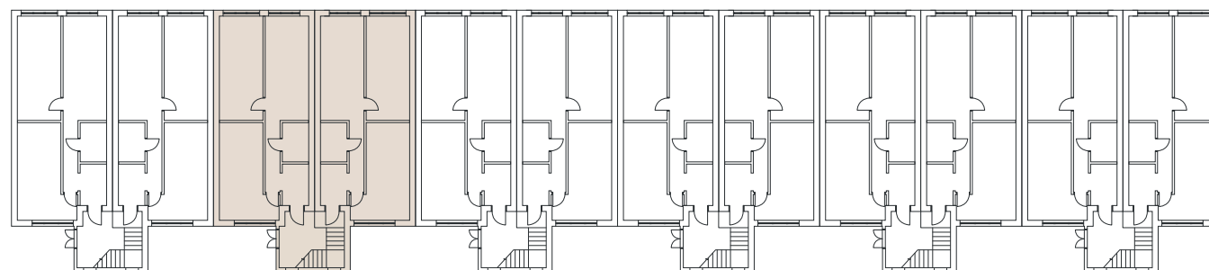
План первого этажа
